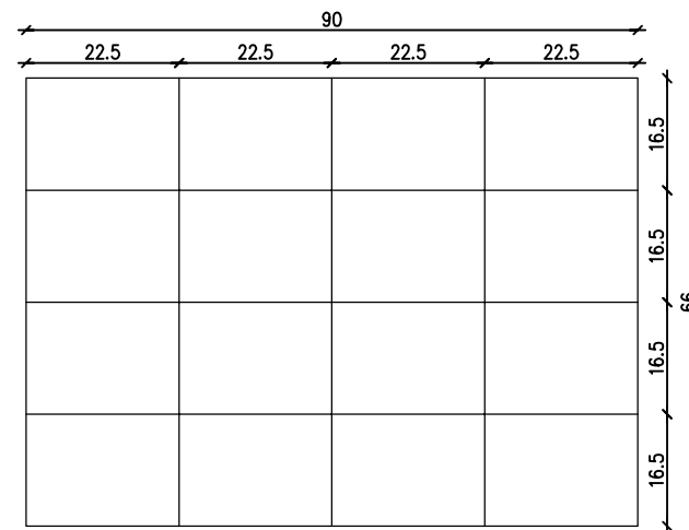
Zbrojenie do płyty \varnothing 8
