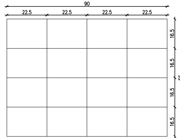
Zbrojenie do płyty \varnothing 6
