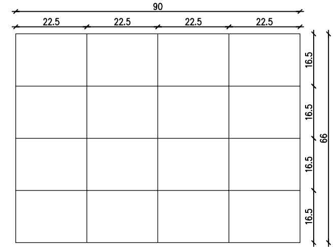
Zbrojenie do płyty \varnothing 8
